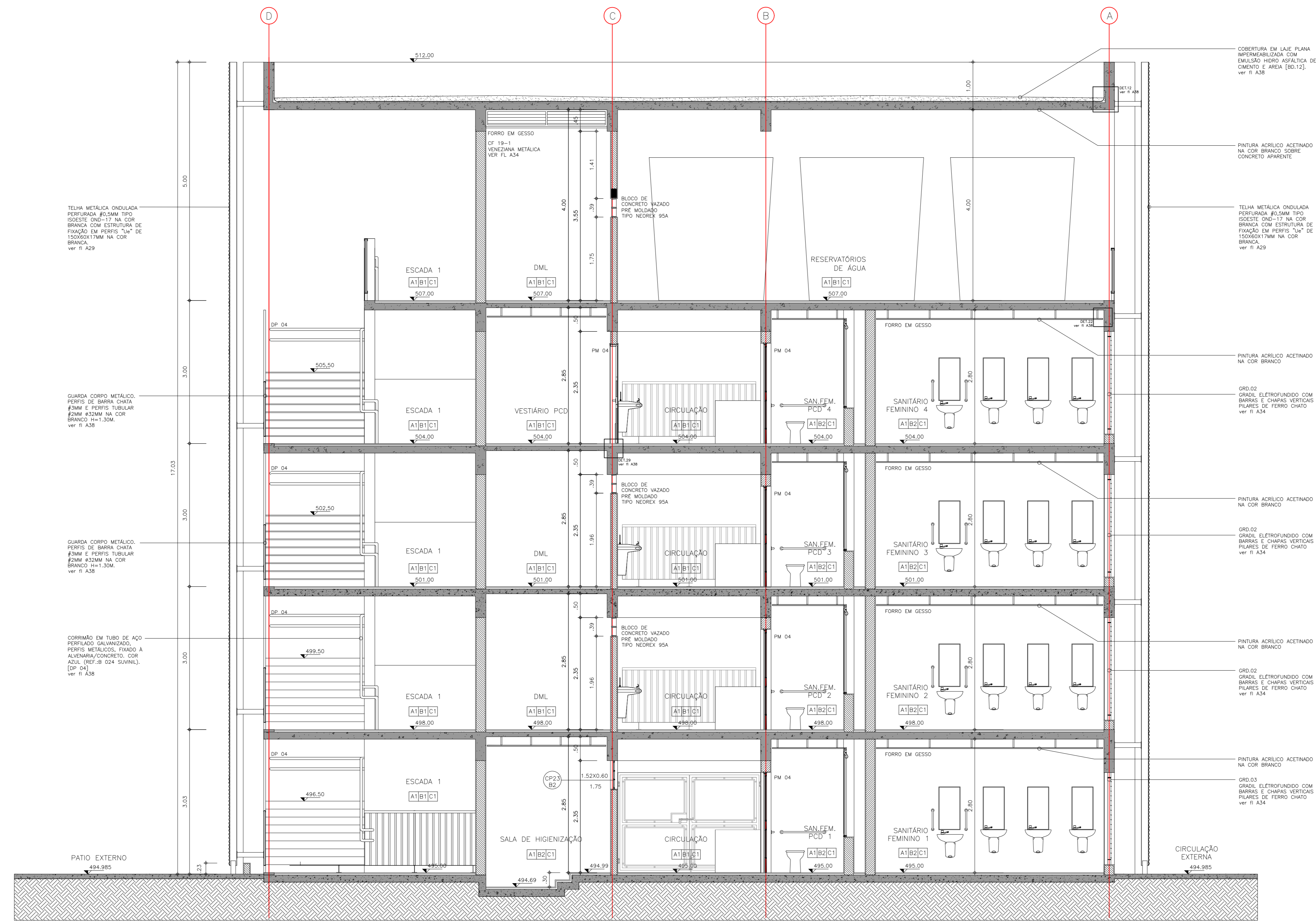
CORTE DD ESCALA 1:30
